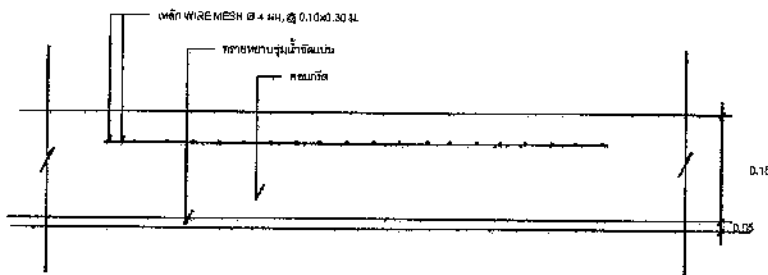
รายละเอียดถนนคอนกรีตเสริมเหล็ก
