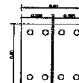
ขยายหน้าบ่อพักคอนกรีต ไม่ใช้ปูนทราย
