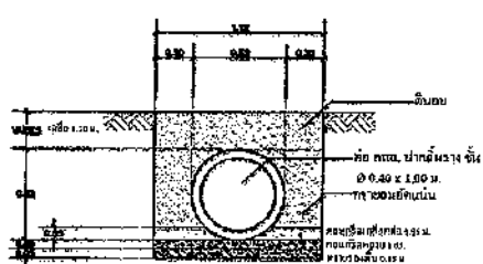
รูปตัด ๐๐ ขยาย ๑:๑๐
