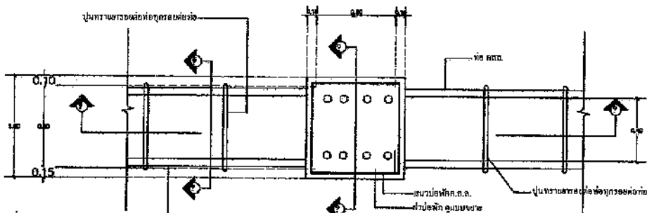
แปลนและหน้าบ่อพักขยายหน้าบ่อพัก ไม่ใช้ปูนทราย
