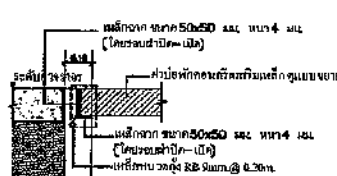
รูปขยายหน้าบ่อพัก ไม่ใช้ปูนทราย
