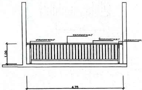
ขยายราวสแตนเลส(2)
