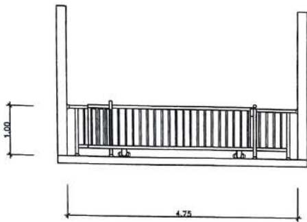
ขยายราวสแตนเลส (A) มาตราส่วน 1:75
