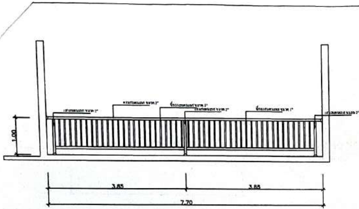
ขยายราวสแตนเลส(1)
